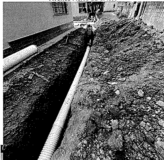
CONSERVACION SISTEMA DE ALCANTARILLADO SANITARIO Y PLUVIAL AREA URBANA (2024), COBAN, ALTA VERAPAZ SNIP 322919 Avance Físico de 8.43%
